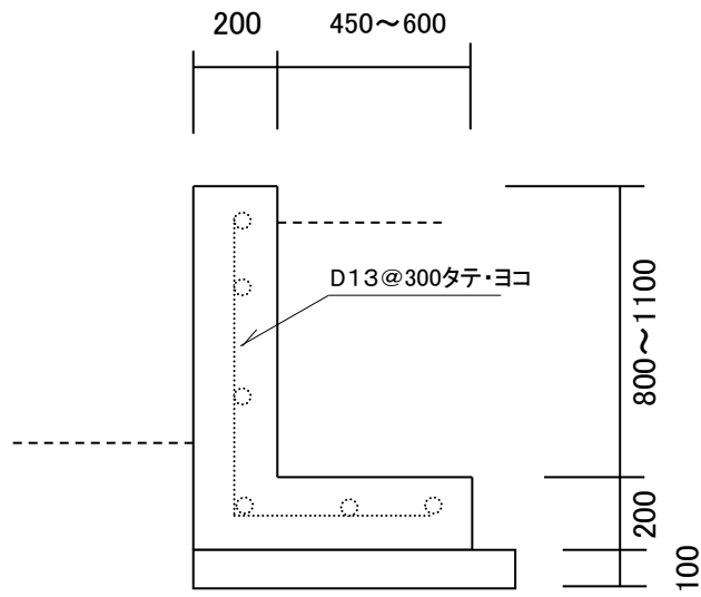
① L型擁壁工 延長 9.04m
