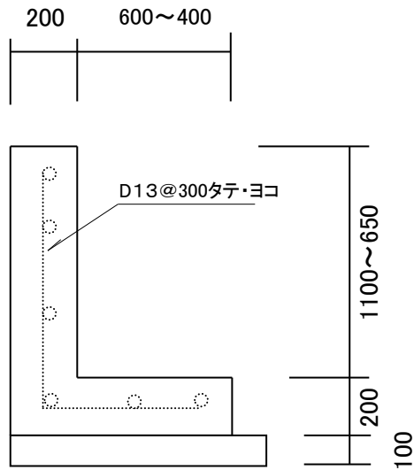
② L型擁壁工 延長 4.0m
