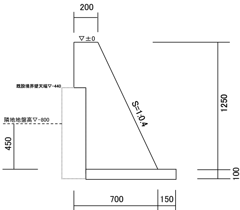
①重力式擁壁工 L=13.2m
