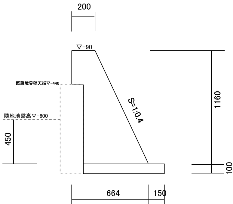
②重力式擁壁工 L=2.8m
