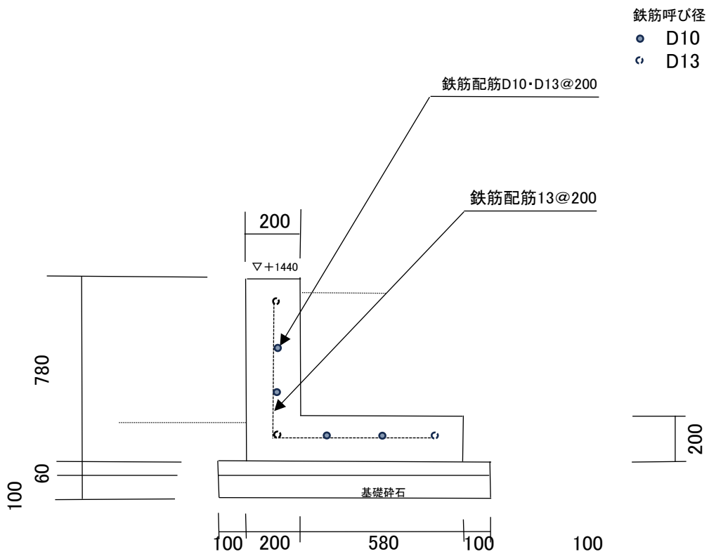
④ L型擁壁工 L=7.8m
