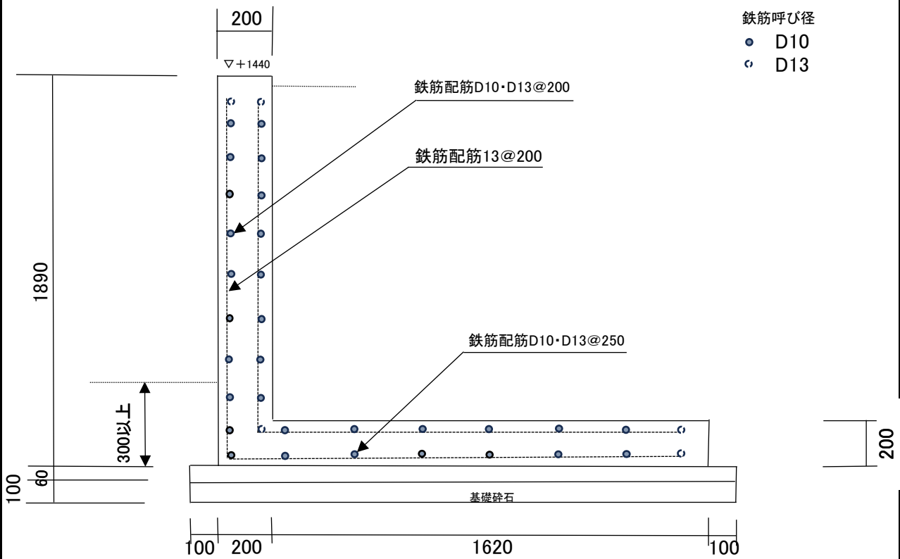
④ L型擁壁工 L=7.8m
